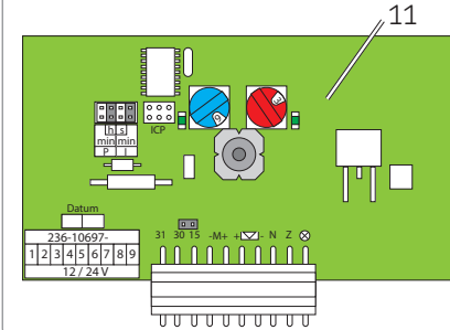
Pletina de mando quitada Fig. 23
