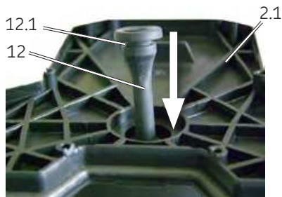
Montar el tubo flexible de drenaje Fig. 24
