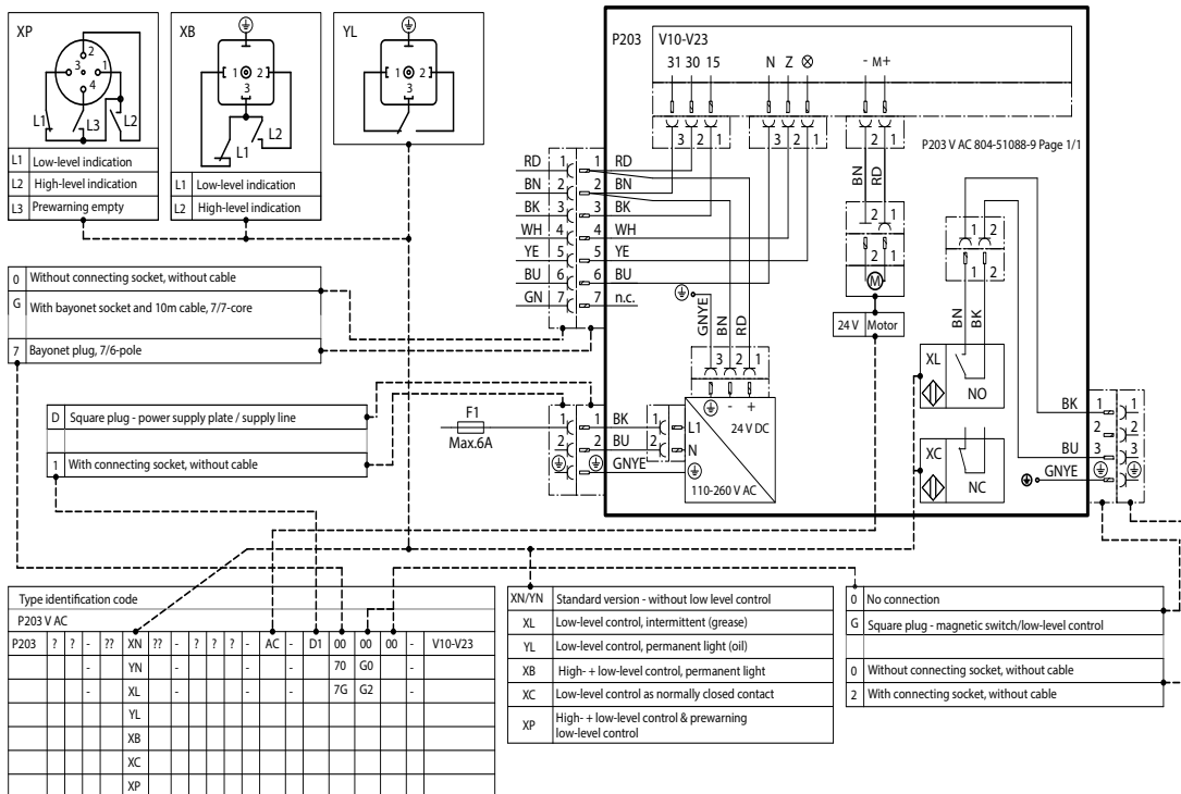
Esquema de conexiones P203 V AC con pletina de mando V Fig. 44
