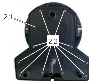
Montar la tapa de la carcasa Fig. 26
