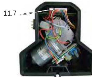
Enchufe de la pletina de mando Fig. 22
